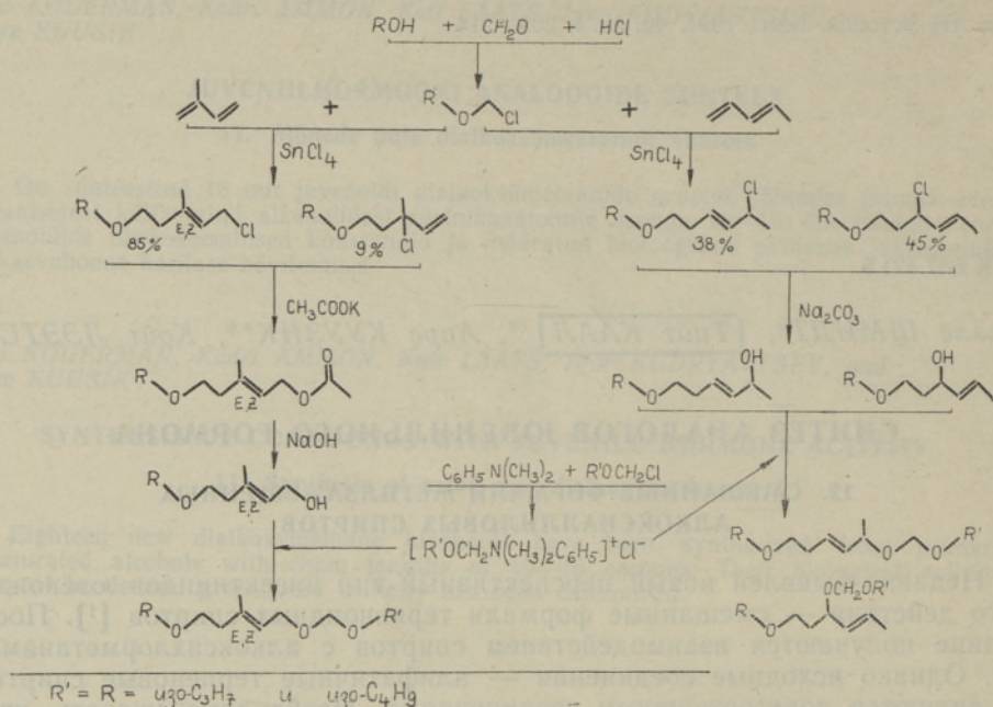
Схема синтеза смешанных формалей метилзамещенных алкоксиаллиловых спиртов
